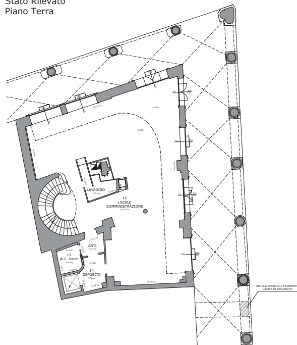
Stato Rilevato Piano Terra
