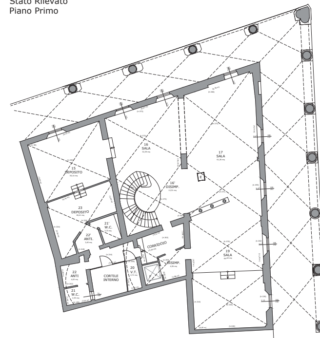
Stato Rilevato Piano Primo
