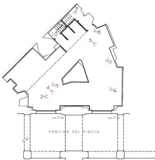
STATO ATTUALE PIANO TERRA
