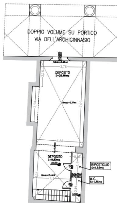
PIANTA PIANO AMMEZZATO
